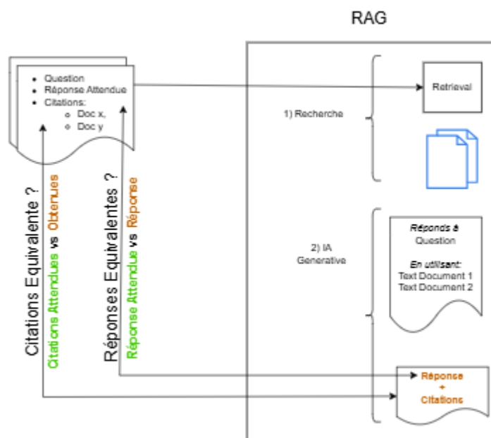
Figure 7 : Éléments constitutifs de l'évaluation double d'une chaîne de RAG
