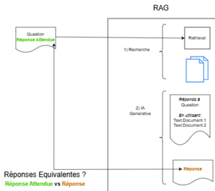
Figure 4 : Éléments constitutifs de l'évaluation simple d'une chaîne de RAG
