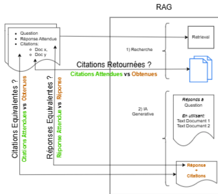
Figure 8 : Éléments constitutifs de l'évaluation triple d'une chaîne de RAG
