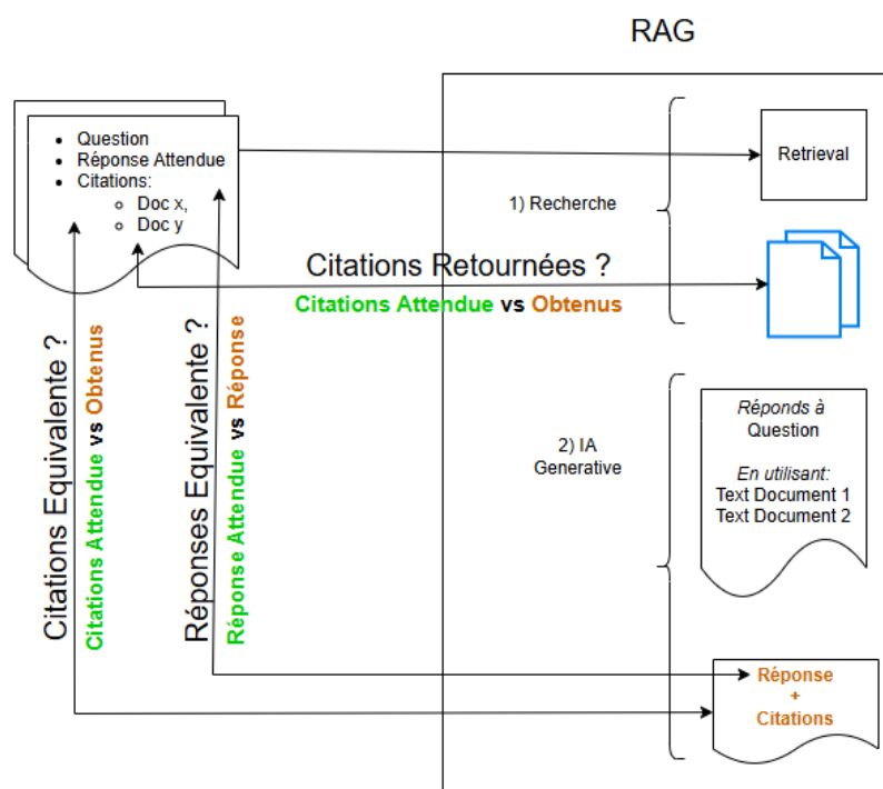
Figure 9 : Schéma RAG citations retournées
